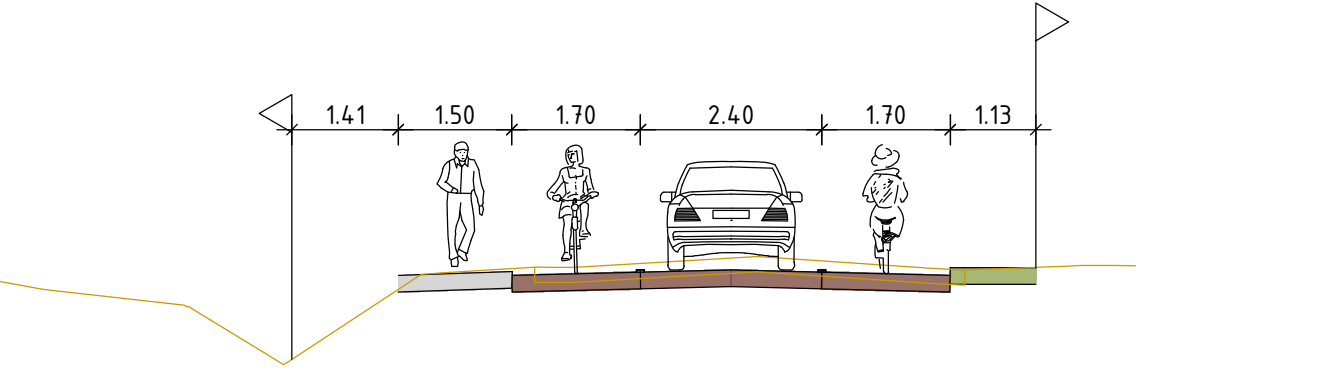
Normaalprofiel binnen bebouwde kom
