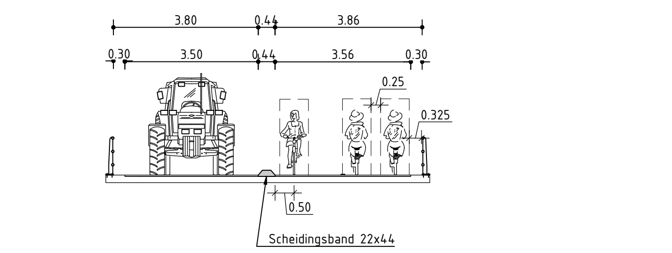
Profiel om-en-om-regeling viaduct A15
